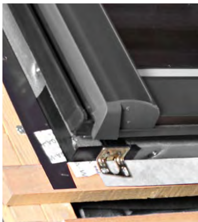
Wykonanie uszczelnienia wodoodporną taśmą dookoła okna.
