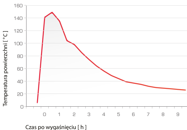
Piecyk kominkowy z akumulacją
